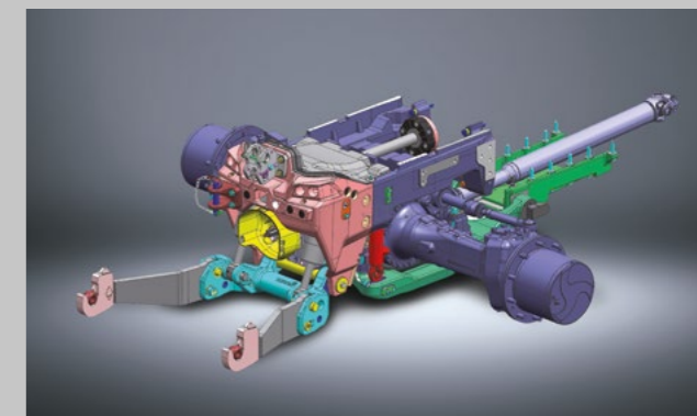
Elektronicky ovládané odpružení přední nápravy se systémem kontroly stability a polohy. Systém odpružení je možné používat jak při přepravě, tak v těžkém tahu. V případě potřeby je možné systém zcela odpojit.
